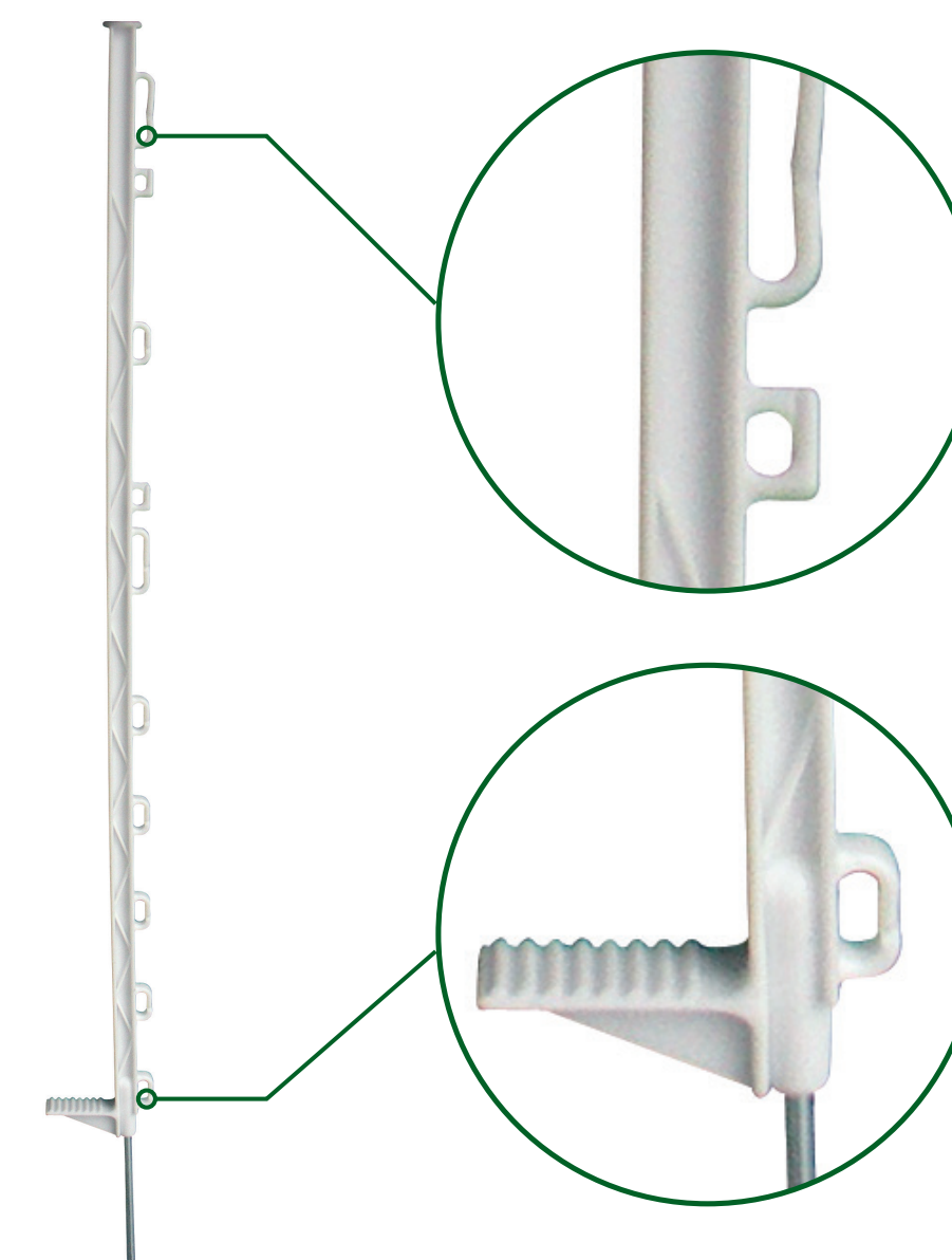
Palica za pastirja 105 cm z izolatorji
